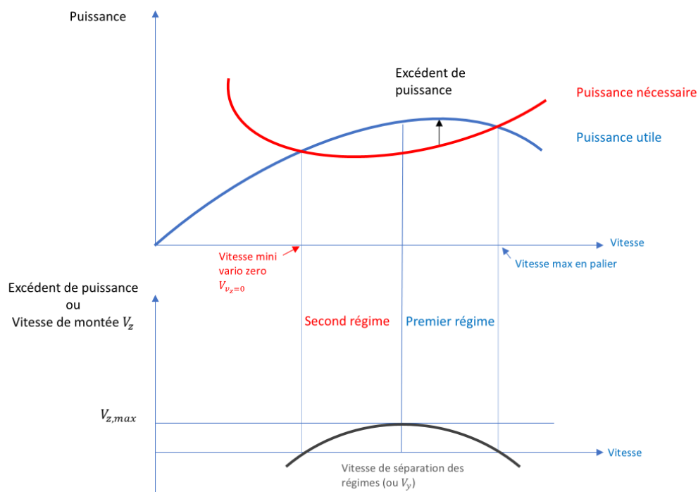
Figure 6 : régimes de vol d'un avion à altitude densité importante (Source : BEA)
