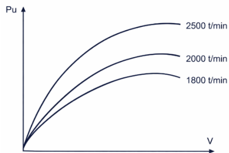
Figure 3 : courbe de puissance utile à différents régimes moteur avec une hélice à calage fixe
