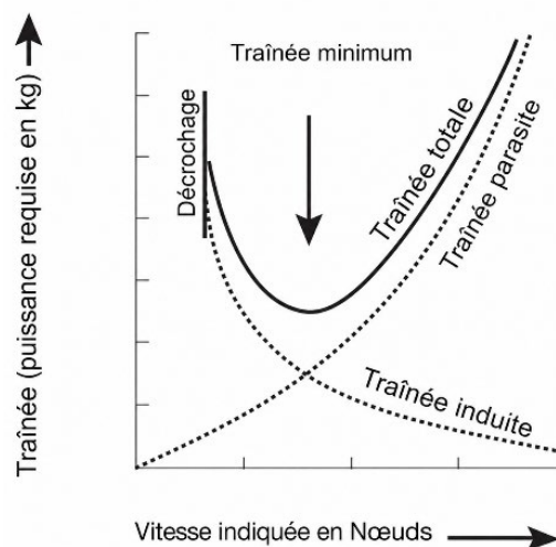
Figure 2 : évolution de la traînée en fonction de la vitesse air 1 (source : ENAC)
