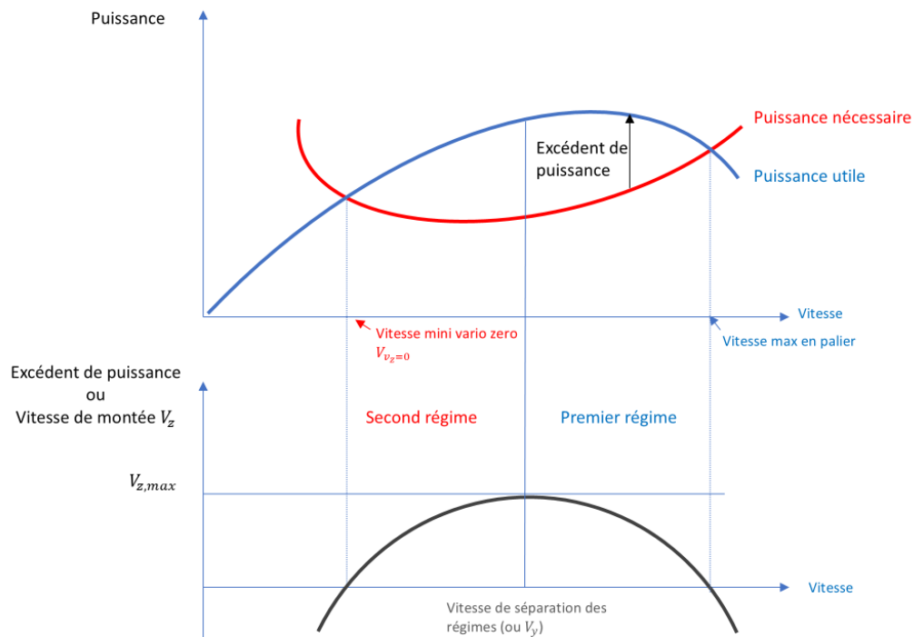
Figure 5 : régimes de vol d'un avion à une faible altitude densité (Source : BEA)
