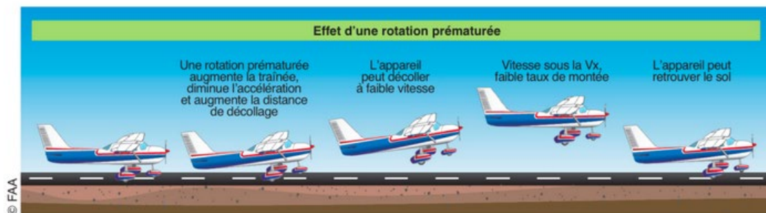
Figure 8 : illustration de l'effet d'une rotation prématurée (Source : FAA, traduction BEA)
