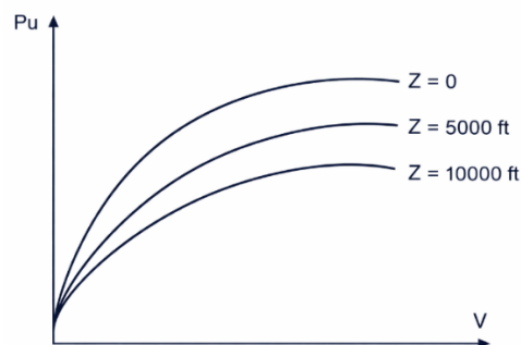
Figure 4 : courbe de puissance utile en fonction de l'altitude pression avec une hélice à calage fixe
